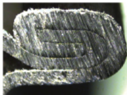
上海弗列加滤清器咬口处之微照。
