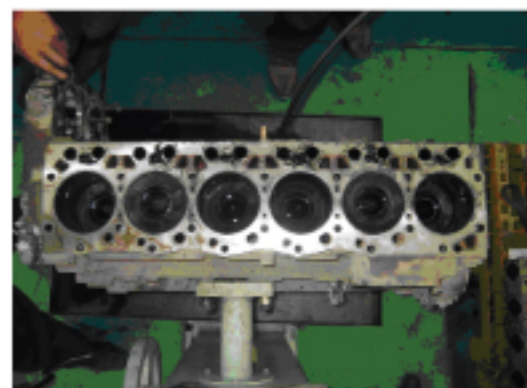
发动机缸套磨损情况
