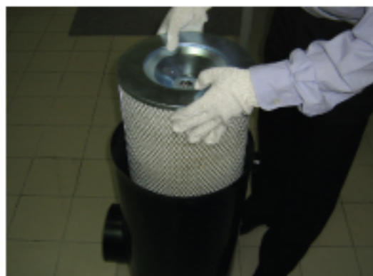
3.小心拿出主滤芯
