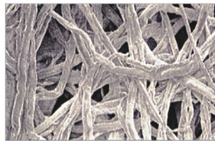
一般滤清器用的粗劣滤纸。
