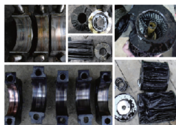
机油滤清器芯破裂导致轴瓦损坏
