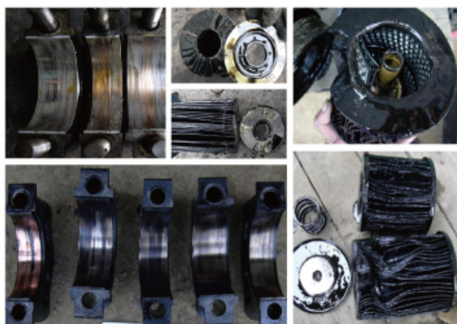
机油滤清器芯破裂导致轴瓦损坏
